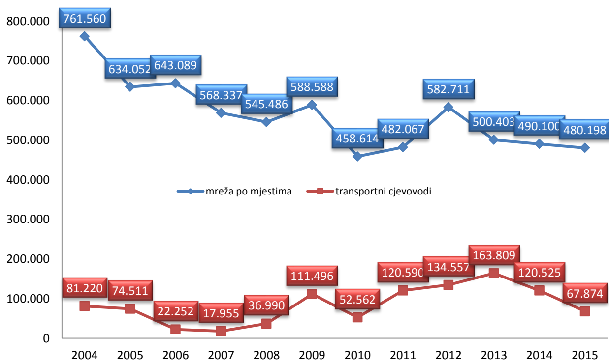
SLIKA: GUBICI NA VODOOPSKRBNOM SUSTAVU MREŽNI I TRANSPORTNI CJEV.
