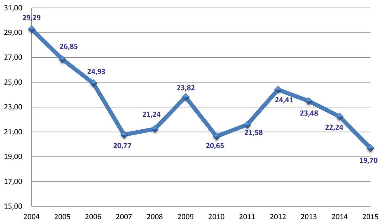
SLIKA: GUBICI NA VODOOPSKRBNOM SUSTAVU (%)
