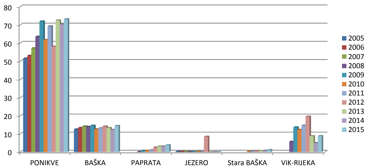
SLIKA: ZAHVAĆENE I PREUZETE KOLIČINE VODE – PROSJEČNO l/s/dan
