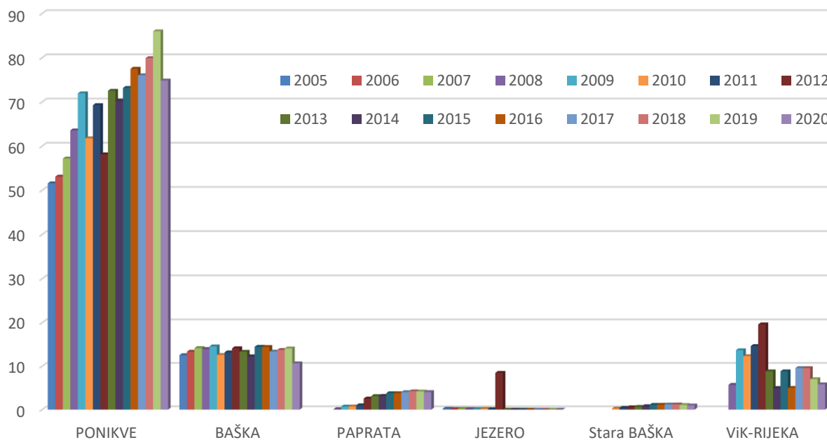
SLIKA: ISPORUČENA (PROČIŠĆENA) KOLIČINA VODE ZA PIĆE – PROSJEČNO l/s/dan
